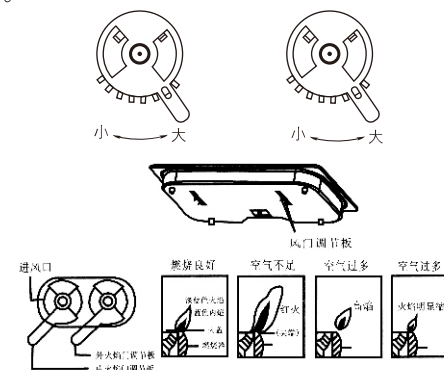
风门调节示意图
